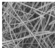
平均繊維径約7～8ミクロン グラスウール10K
