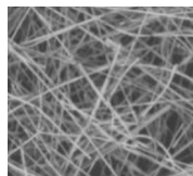
平均繊維径約5～6ミクロン
